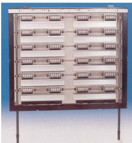
Châssis porte-numérateurs de deux arrêts extérieurs avec ressort de retour.
