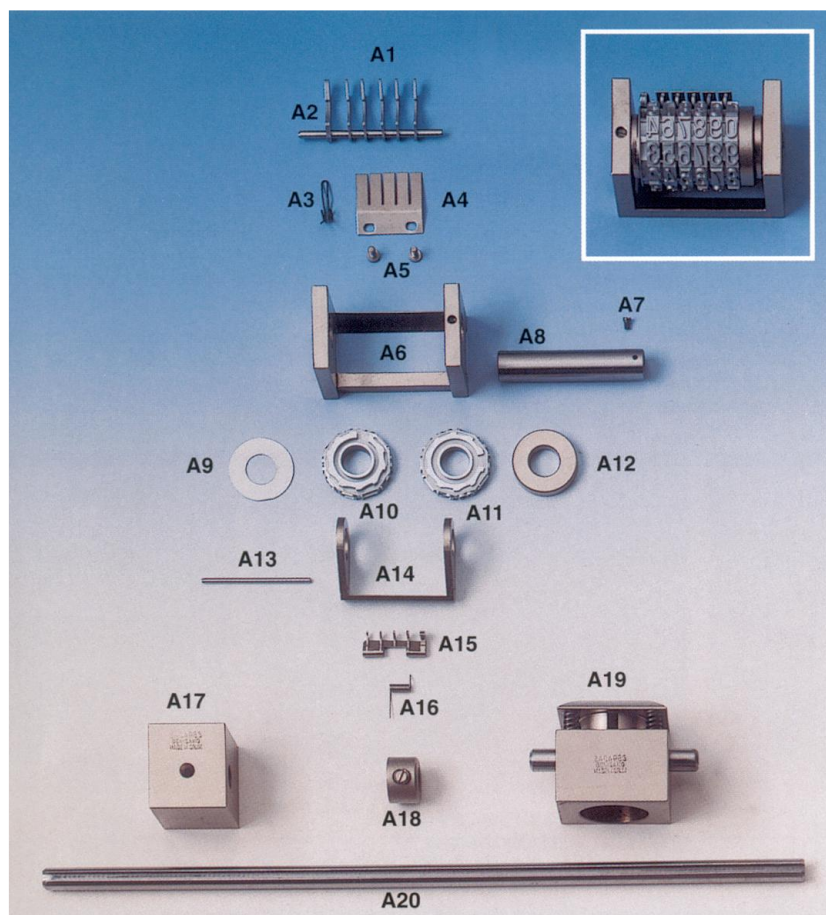
Numéroteur à commande centrale, 6 molettes, gothique 4,5 mm. (gravure 0058).
