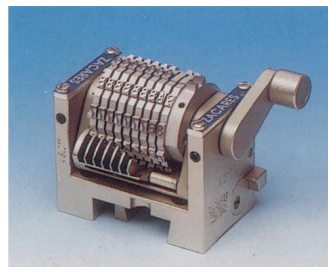
Numéroteur droit à gravure OCR-B1 avec pré-encre et blocage de molettes.
