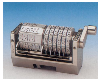
Numéroteur avec gravure spéciale pour loteries.
