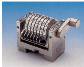
Numéroteur avec gravure arabe.
