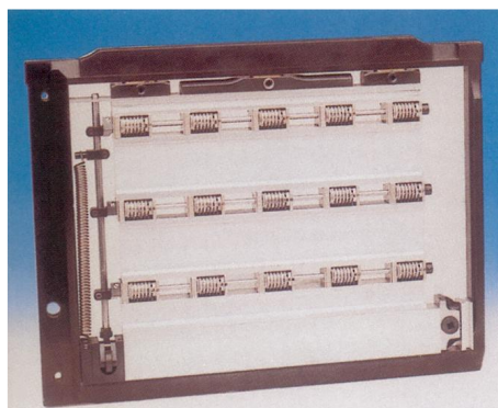
Châssis porte-numérateurs pour machine typographique type Minerva avec changement central à travers le plunger master.
