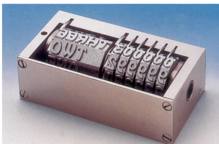
Numéroteur à commande centrale, spécial loteries.
