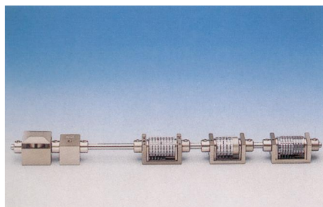
Axe de commande avec rainure montée avec plunger, anneau, ponts et numérateurs.
