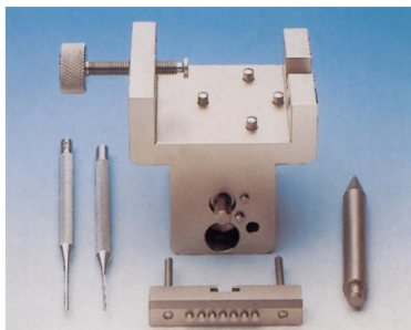
Outil d'assemblage pour les numéroteurs, axe faux et pointeau.
