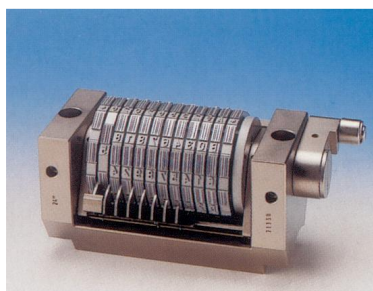
Numéroteur spécial Code-39.
